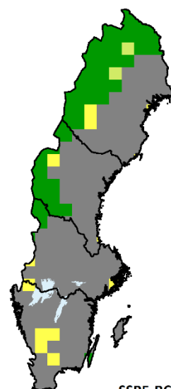
SSP5-RCP8.5
