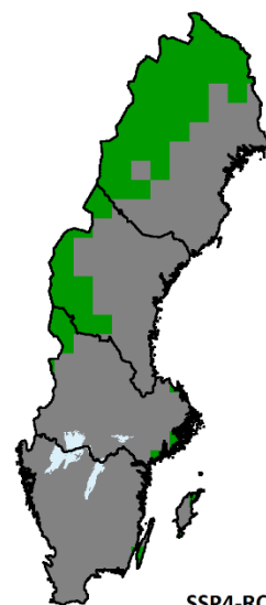
SSP4-RCP4.5
