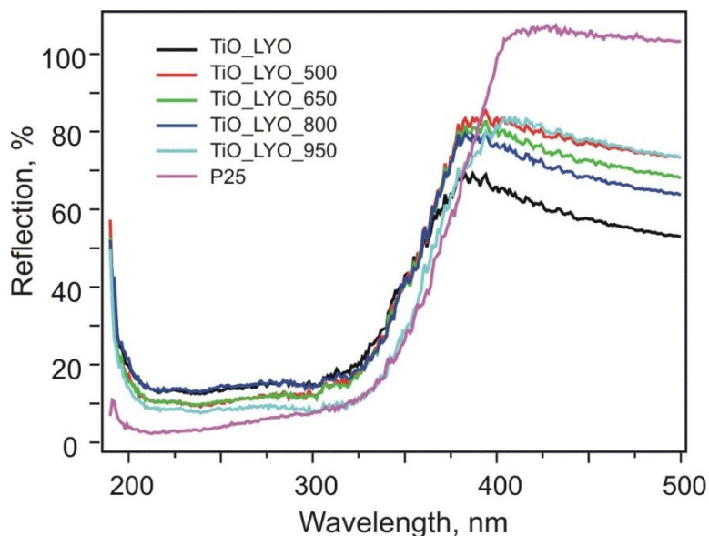
Figure 11. UV-Vis reflection spectra of the samples TiO_LYO, TiO_LYO_500, TiO_LYO_650, TiO_LYO_800 and TiO_LYO_950 and P25
