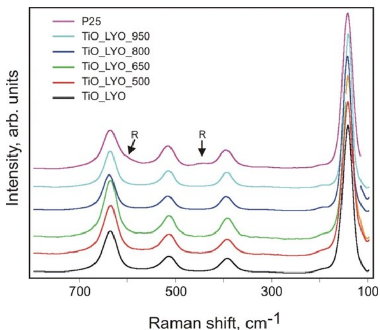
Figure 10. Raman spectra of the samples TiO_LYO, TiO_LYO_500, TiO_LYO_650, TiO_LYO_800 and TiO_LYO_950 and P25.
