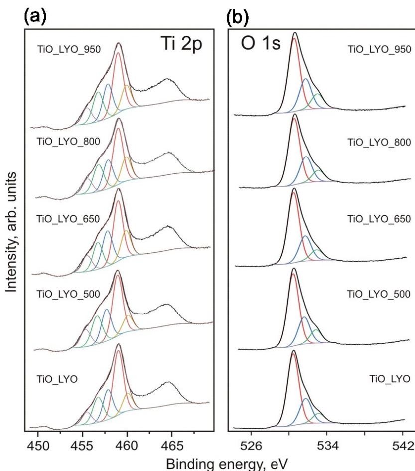
Figure 9. (a) Ti 2p and (b) O 1s XPS spectra of samples TiO_LYO, TiO_LYO_500, TiO_LYO_650, TiO_LYO_800 and TiO_LYO_950.
