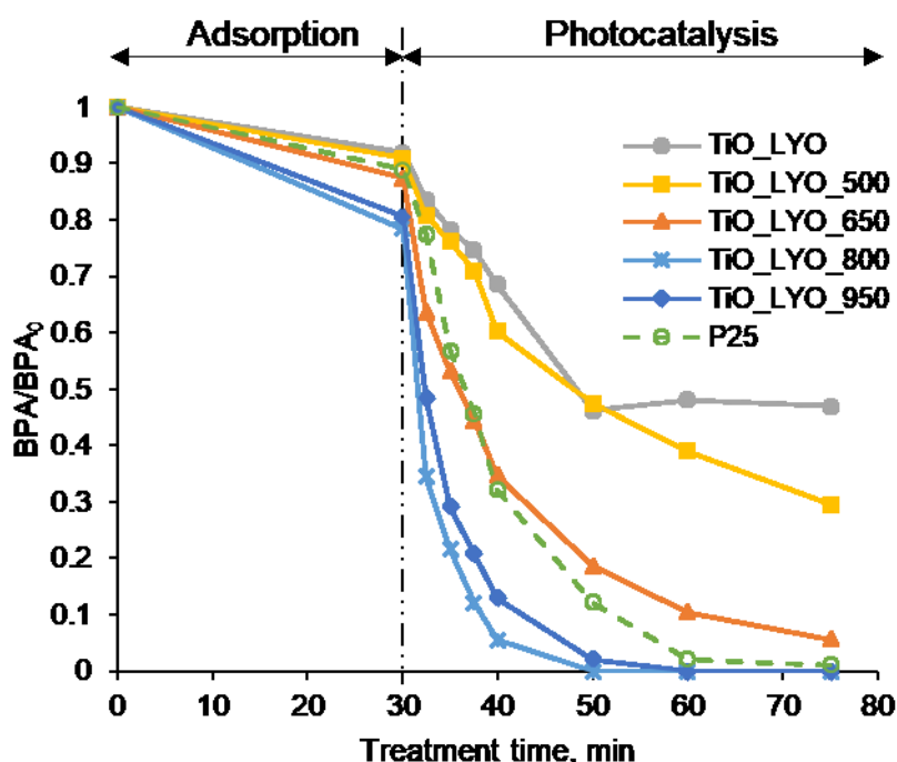
Figure 12. Photocatalytic degradation of BPA in the presence of TiO_LYO, TiO_LYO_500, TiO_LYO_650, TiO_LYO_800, TiO_LYO_950 and Degussa P25 catalysts.
